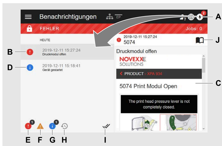
Bild 18: Nach dem Klicken auf das Benachrichtigungs-Symbol (A) öffnet sich die Benachrichtigungs-Ansicht. Die linke Hälfte zeigt die Benachrichtigungs-Historie, die rechte Hälfte zeigt eine Erklärung zum angewählten Eintrag in der Historie.
