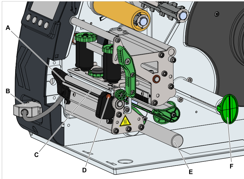
Bild 12: Zusätzliche Bedienteile des XLP 514 mit Spendeoption.
